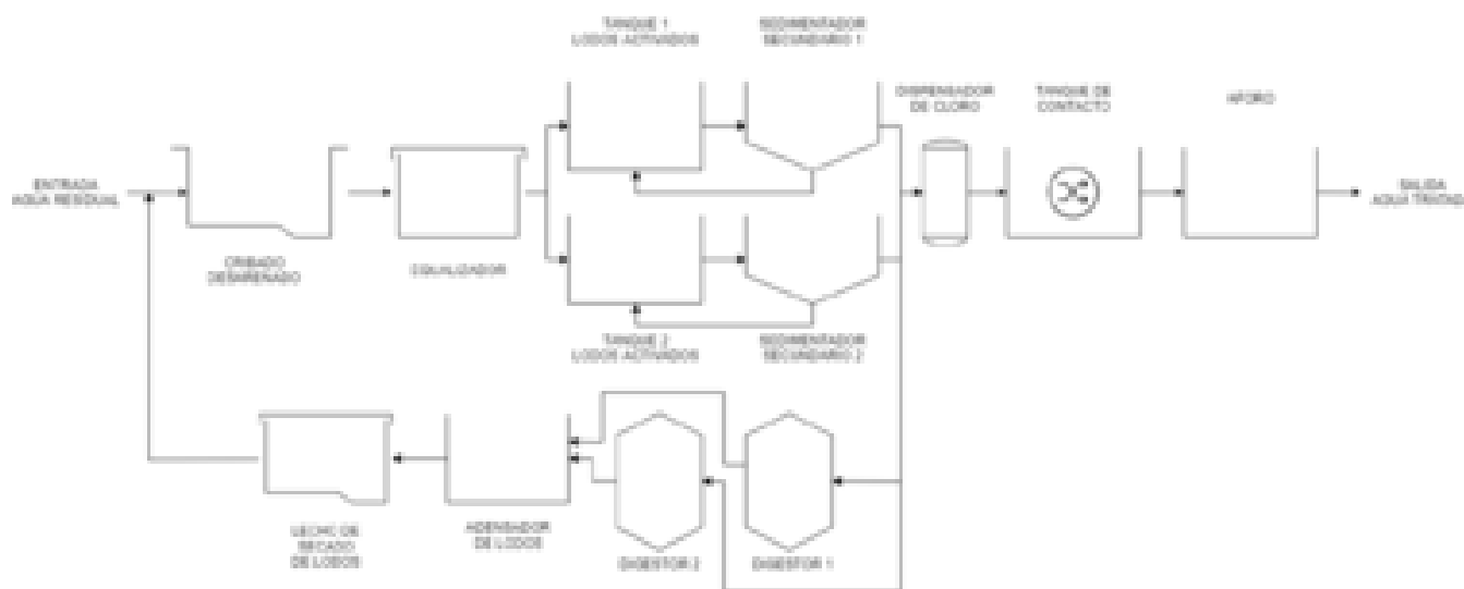
Diagrama del sistema de tratamiento de Finca 3. Fuente: Oficina Ejecutora del Plan de Inversiones (OEPI)
